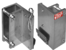
Halteblech Dreibaum/Winde
