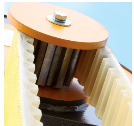
secuwave: Verzahnte Wenderolle und beschichtetes Hebebänder
