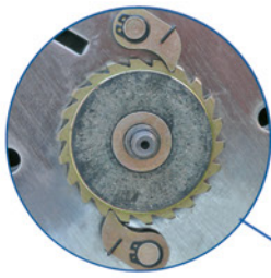
Sicherheitsbremse mit zwei Sperrklinken
